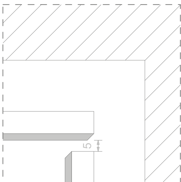
03 Fibrocemento - Angolo interno FBC Internal corner
