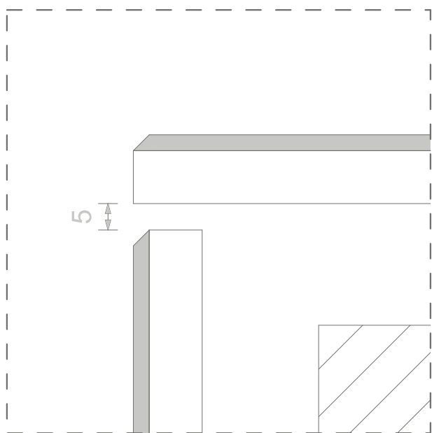
01 Fibrocemento - Angolo esterno FBC External corner
