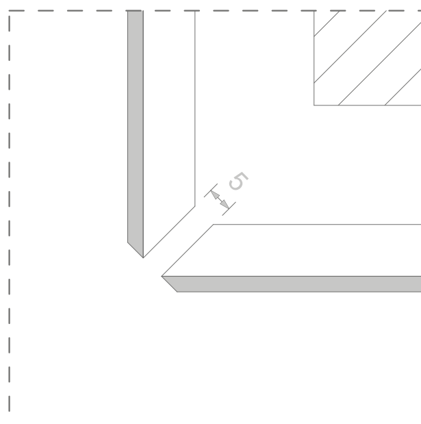
02 Fibrocemento - Angolo esterno con taglio a 45° FBC Mitered cut External corner
